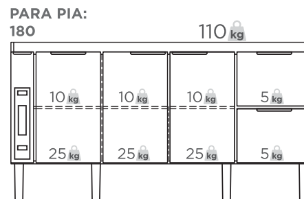
GABINETE L: 174 cm A: 85 cm P: 51 cm
