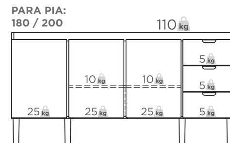
GABINETE L: 174 / 194 cm A: 85 cm P: 51,1 cm
