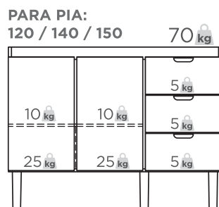
GABINETE L: 114 / 134 / 144 cm A: 85 cm P: 51,1 cm
