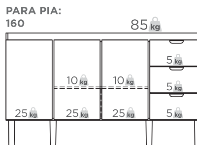
GABINETE L: 154 cm A: 85 cm P: 51,1 cm
