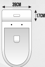
VISTA SUPERIOR CAIXA ACOPLADA RIEDO
